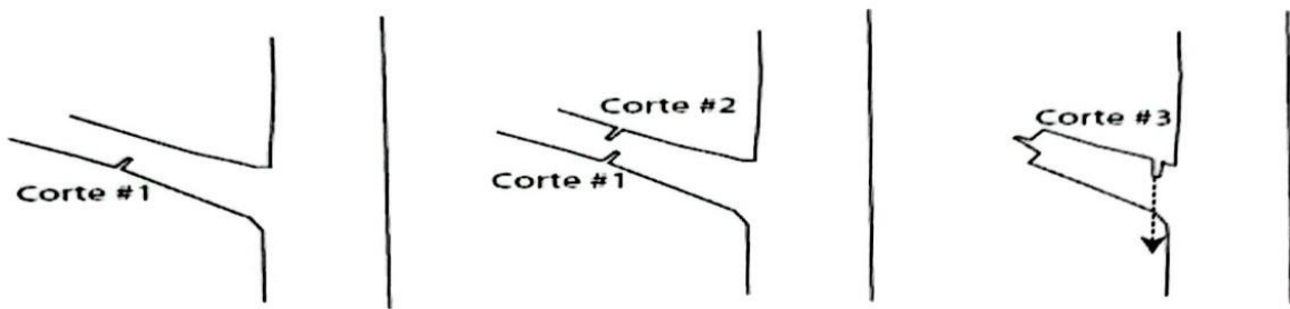
Fig. 1 Pasos para realizar los cortes con motosierra. (Técnica de los 3 cortes).
