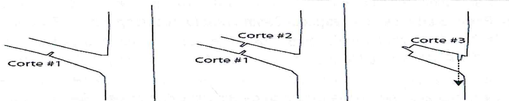
Fig. 1 Pasos para realizar los cortes con motosierra. (Técnica de los 3 cortes).
